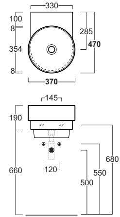
PO 05 Lavabo tondo da appoggio o sospeso Round washbasin wall hung or counter top Ø37.43.h19
