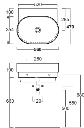
PO 06 Lavabo ovale da appoggio o sospeso Oval washbasin wall hung or counter top 56.43.h19
